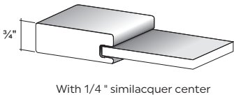
DOOR MODEL BEVERLY 3124 | 45° Assembly
